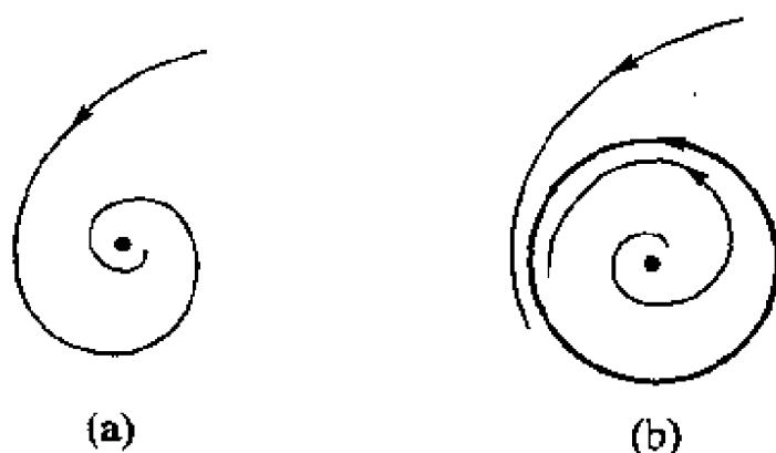
图 8-26 Hopf 分支
