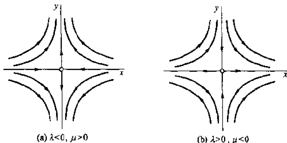
图 8-10 鞍点
